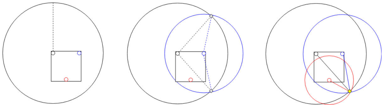
Slika 5 - primjer trilateracije
