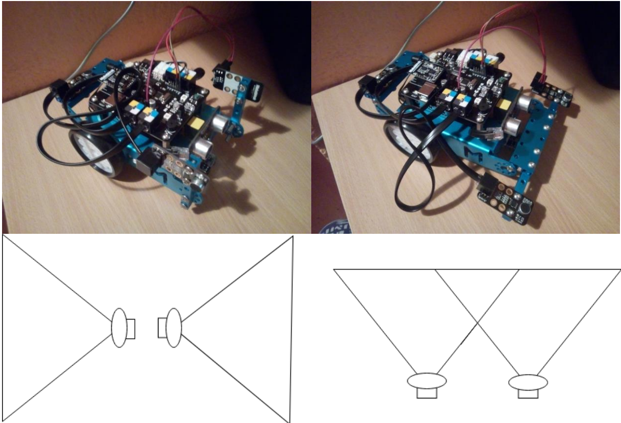
Slika 16 - usporedba područja osjetljivosti vertikalno (slika lijevo) i horizontalno (slika desno) postavljenih senzora zvuka.
