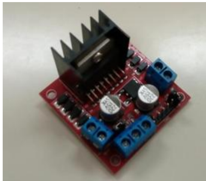
Slika 5 - Priказ L298N Dual H Bridge Motor Controllera
