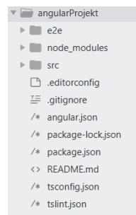
Slika 10. Struktura Angular radnog dijagrama
