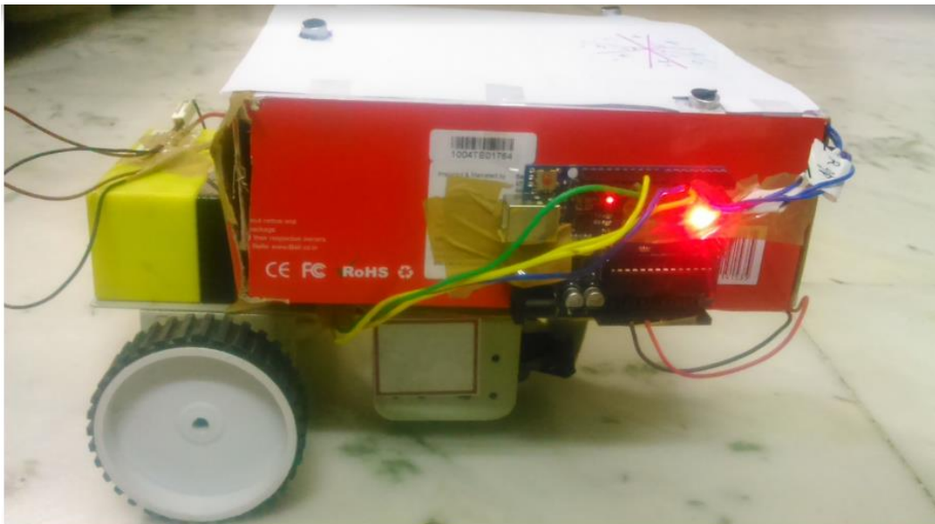
Slika 4 - Blindbot
