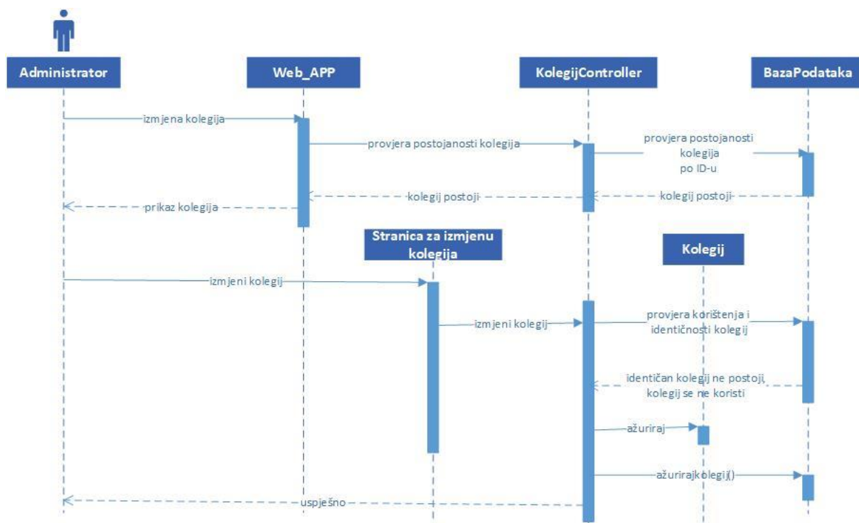
Slika 19. Prikaz sekvencijalnog dijagrama za izmjenu kolegija
