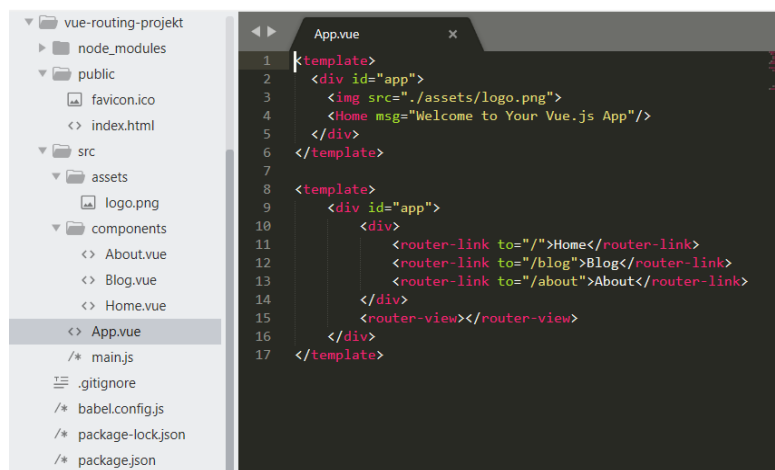
Slika 31. Vue.js linkovi na putanje u predlošku
