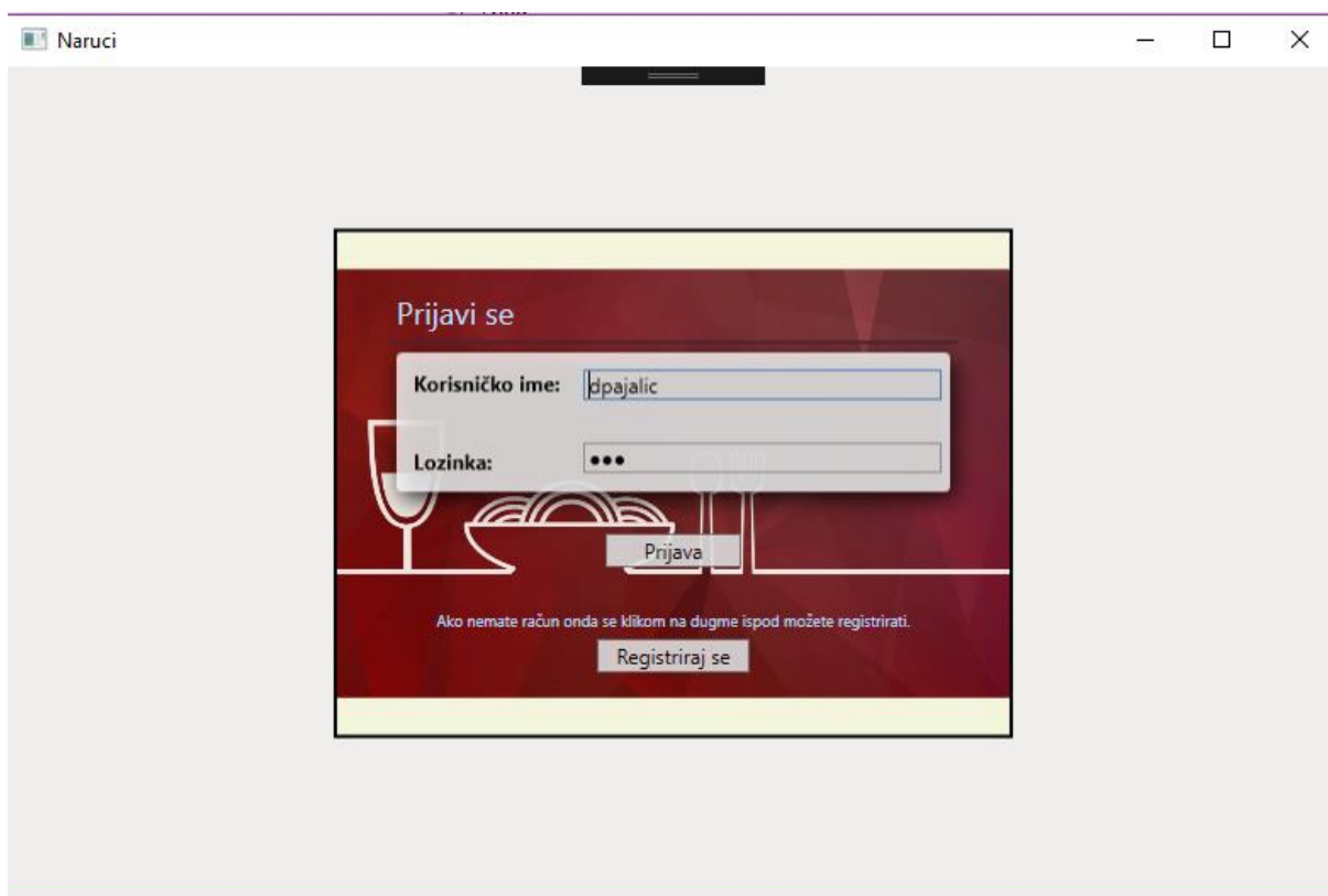
Slika 9 Login
