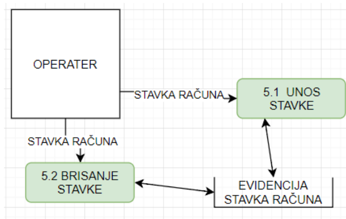
Slika 8. Prikaz dijagrama toka podataka druge razine(Proces 5.)
