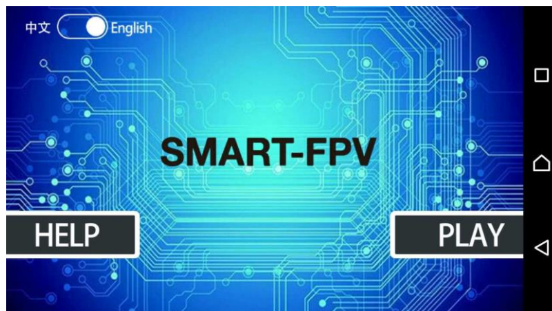
Slika 30.:Sučelje SMART-FPV
