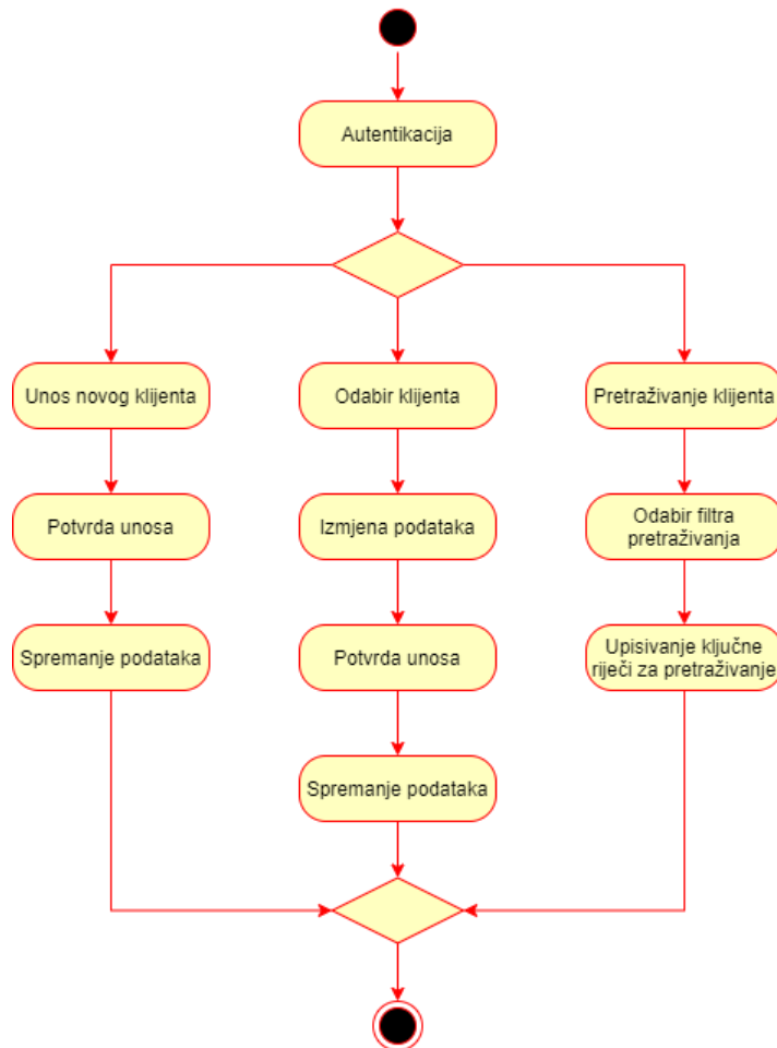
Slika 6 Dijagram aktivnosti za unos novog klijenta
