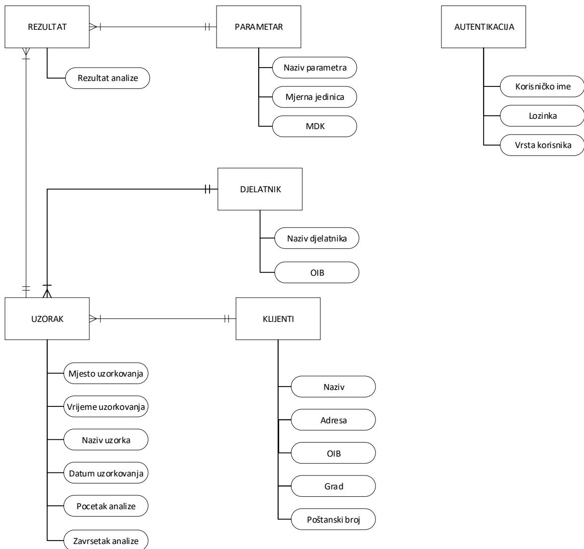
Slika 11 Model entiteti-veze
