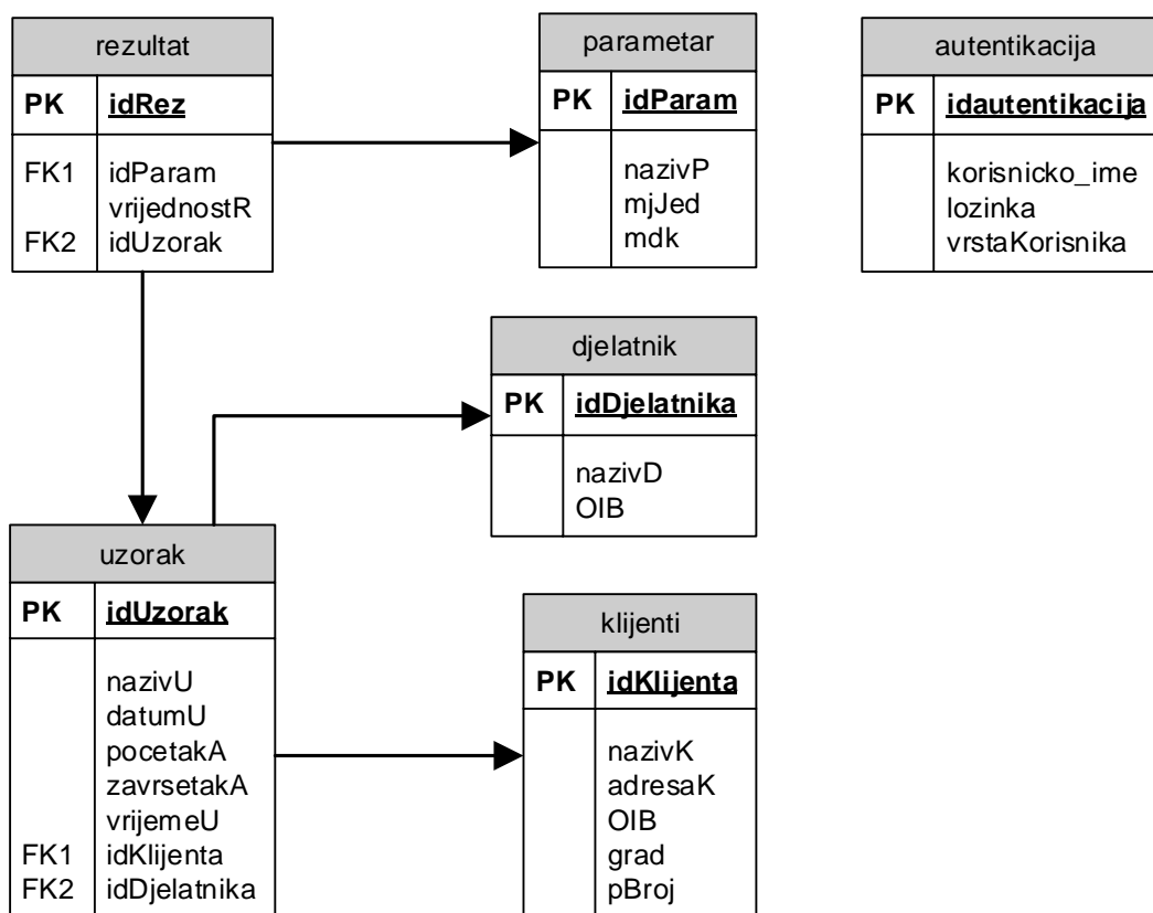
Slika 12 Relacijski model
