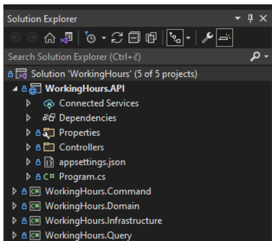
Slika 10 - Struktura API-a
